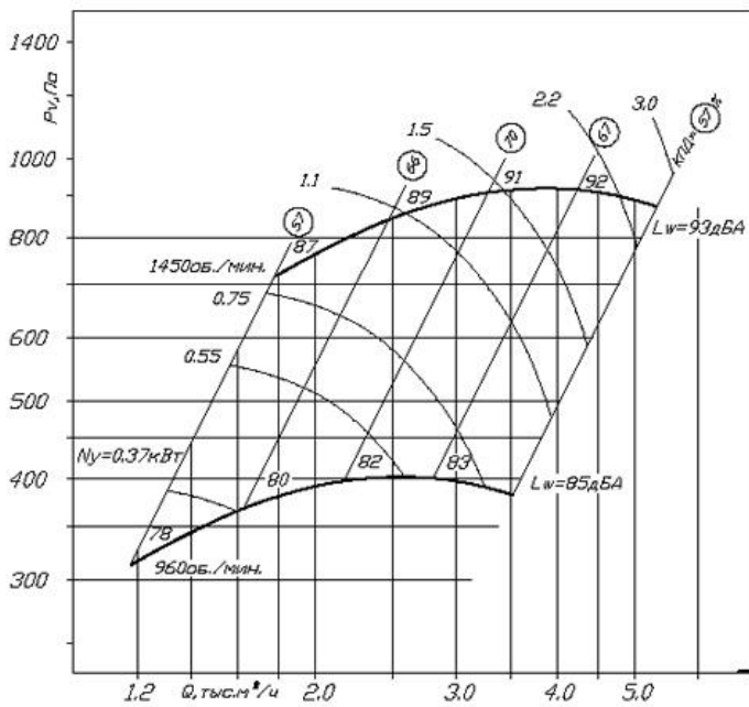
ВЦ 14-46-3.15 схема 1
