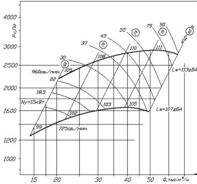
ВЦ 14-46-8 схема 1
