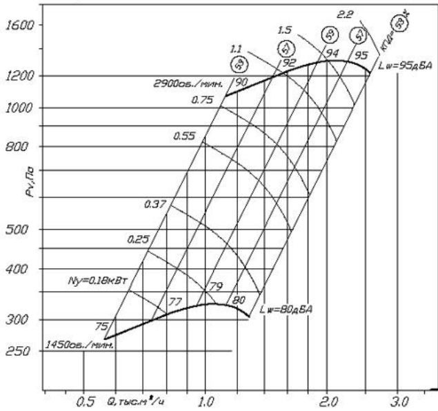
ВЦ 14-46-2 схема 1
