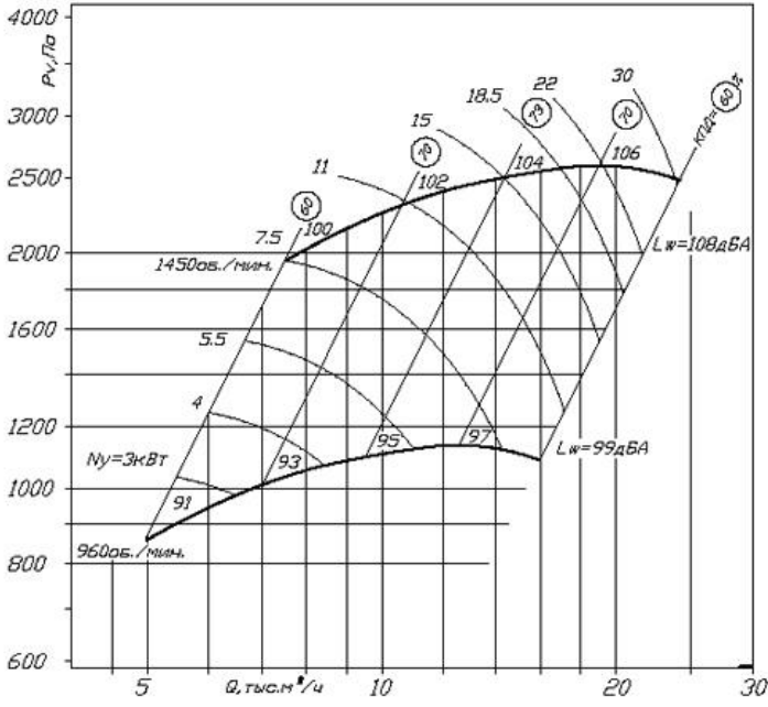
ВЦ 14-46-5 схема 1
