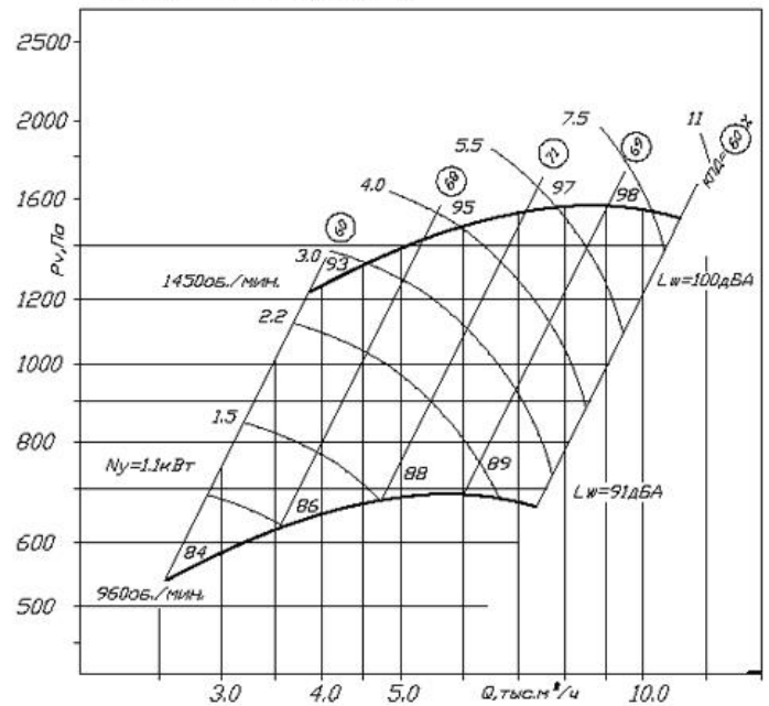
ВЦ 14-46-4 схема 1
