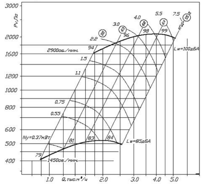
ВЦ 14-46-2.5 схема 1
