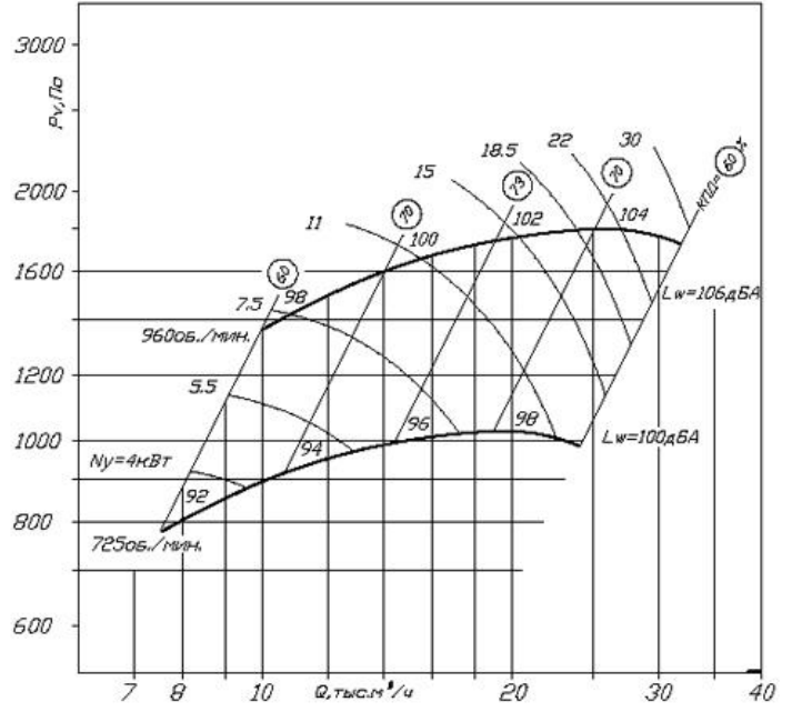
ВЦ 14-46-6.3 схема 1
