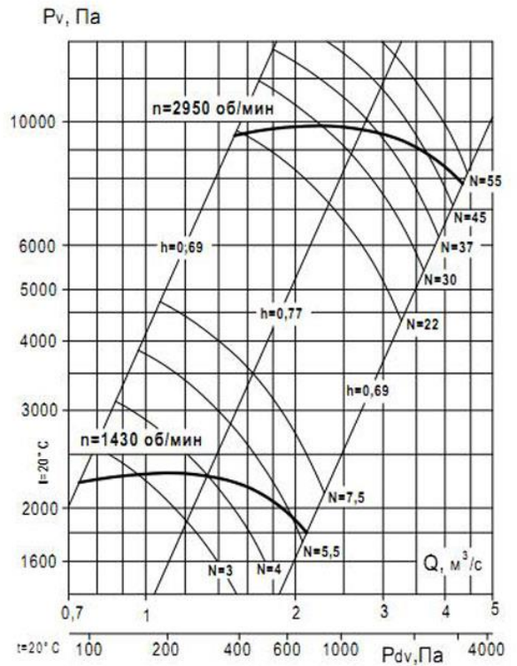
Аэродинамическая характеристика вентилятора ВР 132-30 №7,1 (1 исполнение)
