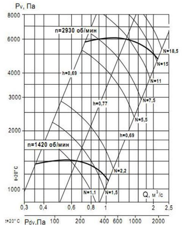
Аэродинамическая характеристика вентилятора ВР 132-30 №5,6 (1 исполнение)
