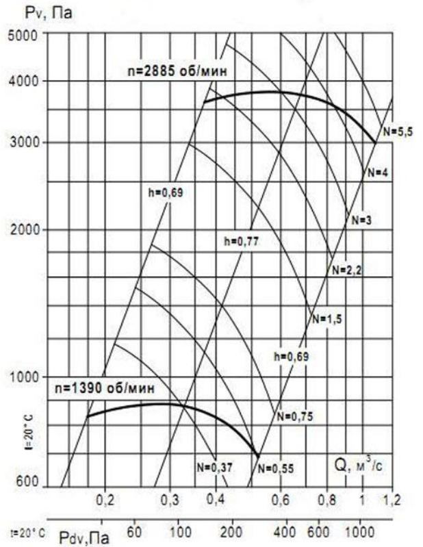
Аэродинамическая характеристика вентилятора ВР 132-30 №4,5 (1 исполнение)
