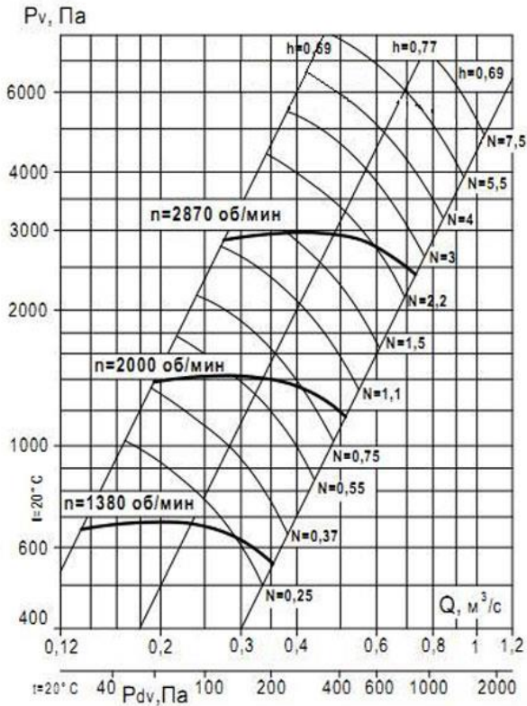
Аэродинамическая характеристика вентилятора ВР 132-30 №4 (1 и 5 исполнение)
