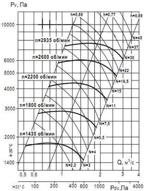
Аэродинамическая характеристика вентилятора ВР 132-30 №6,3 (1 и 5 исполнение)
