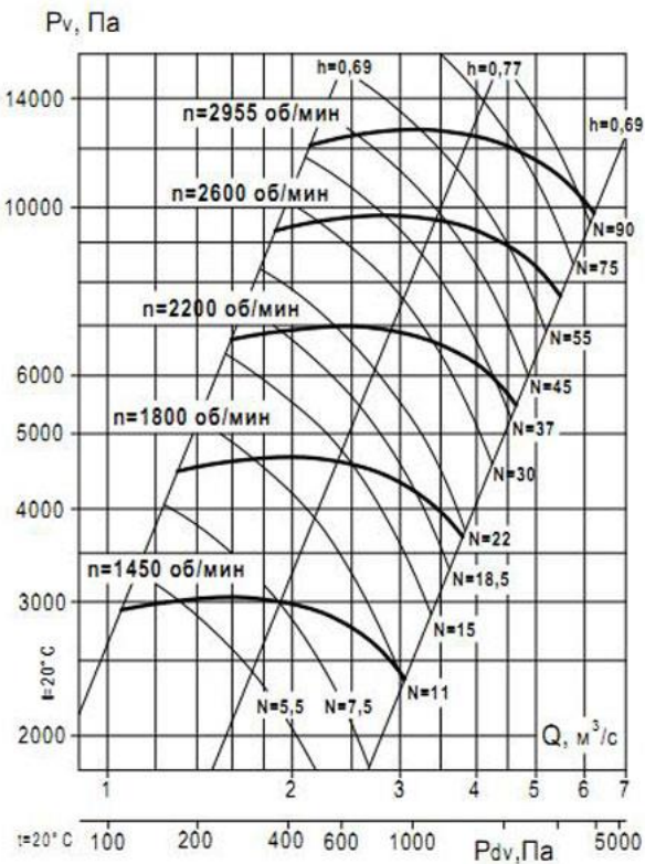
Аэродинамическая характеристика вентилятора ВР 132-30 №8 (1 и 5 исполнение)
