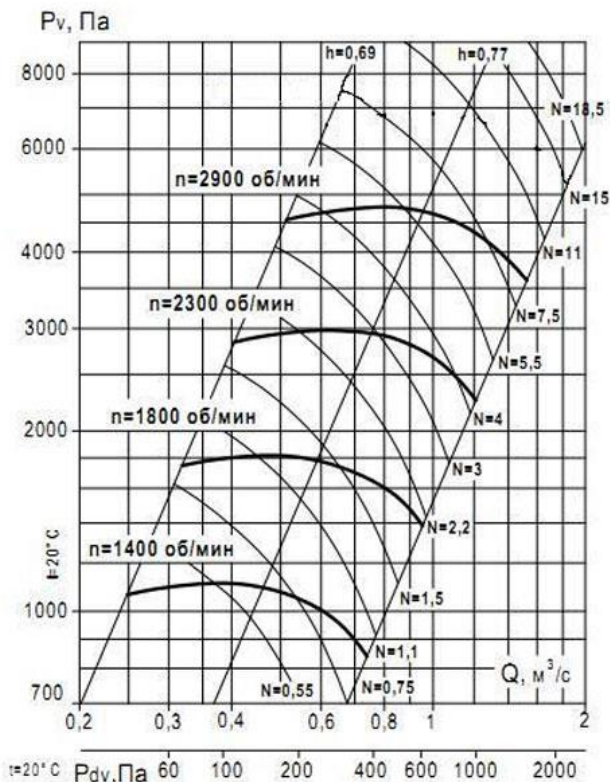
Аэродинамическая характеристика вентилятора ВР 132-30 №5 (1 и 5 исполнение)
