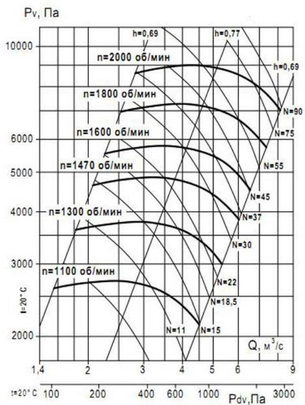
Аэродинамическая характеристика вентилятора ВР 132-30 №10 (1 и 5 исполнение)
