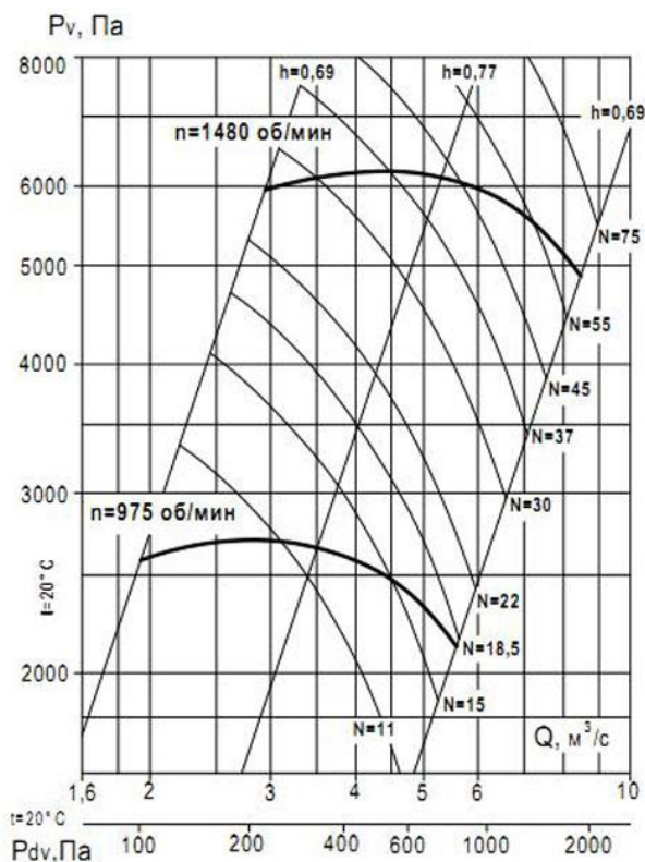
Аэродинамическая характеристика вентилятора ВР 132-30 №12,5 (1 и 5 исполнение)
