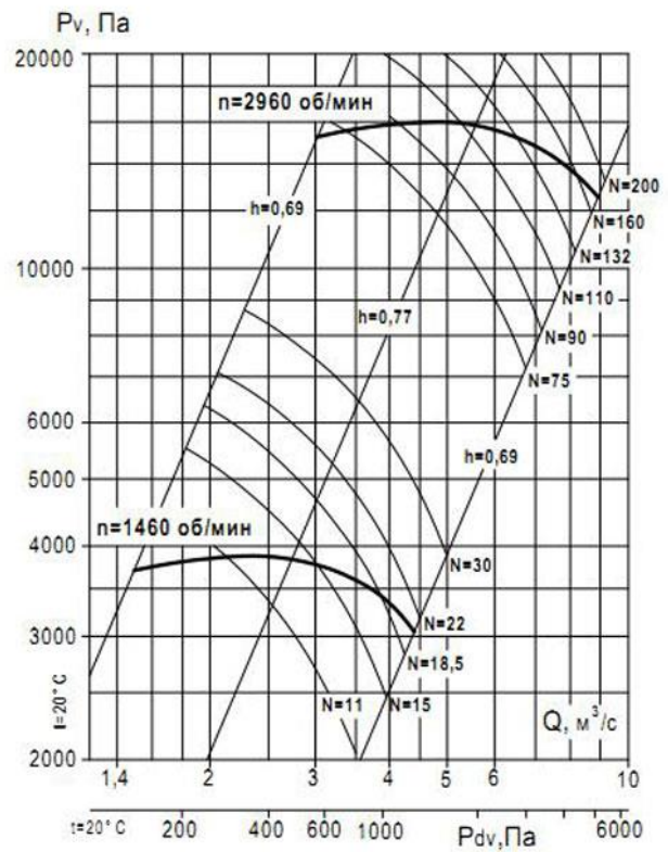
Аэродинамическая характеристика вентилятора ВР 132-30 №9 (1 исполнение)
