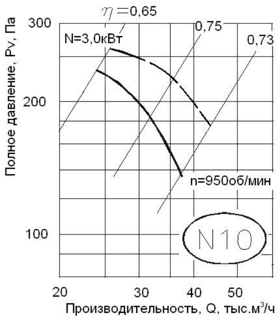
Аэродинамическая характеристика вентилятора ВО 06-300 №10
