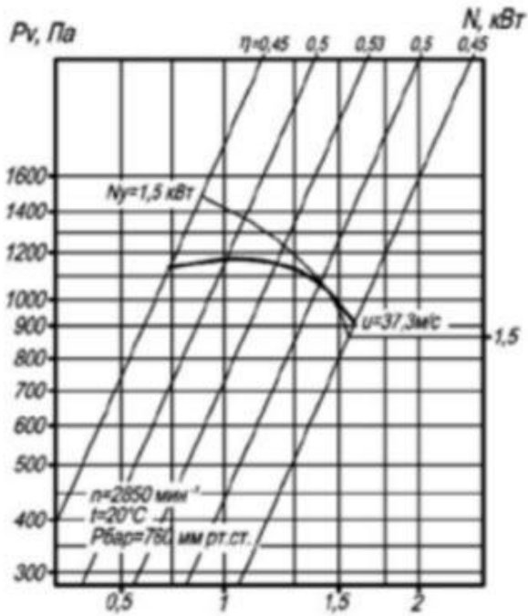
Аэродинамическая характеристика вентилятора ВЦП 7-40 №2,5 схема 1
