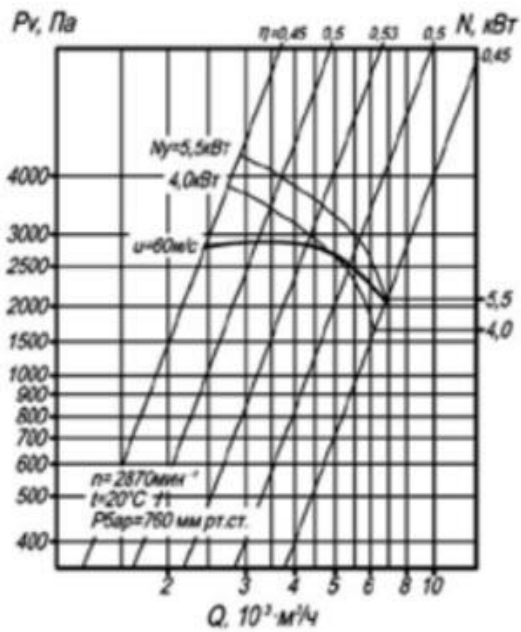
Аэродинамическая характеристика вентилятора ВЦП 7-40 №4 схема 1
