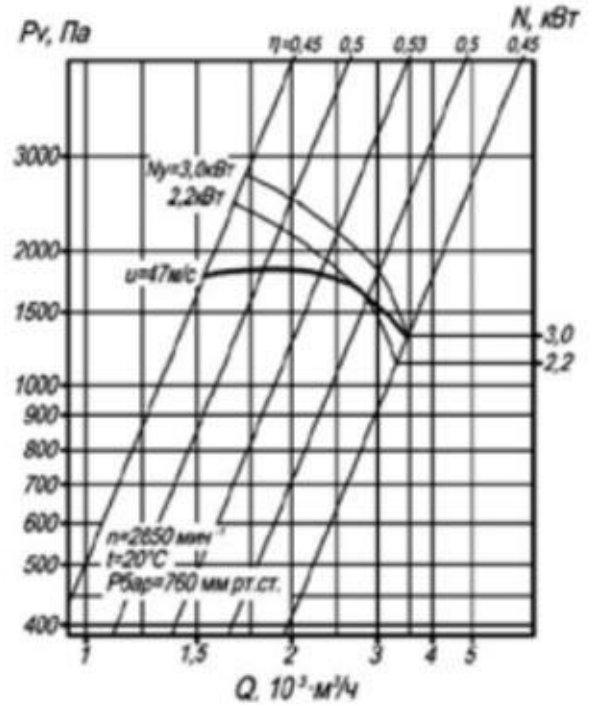
Аэродинамическая характеристика вентилятора ВЦП 7-40 №3,15 схема 1
