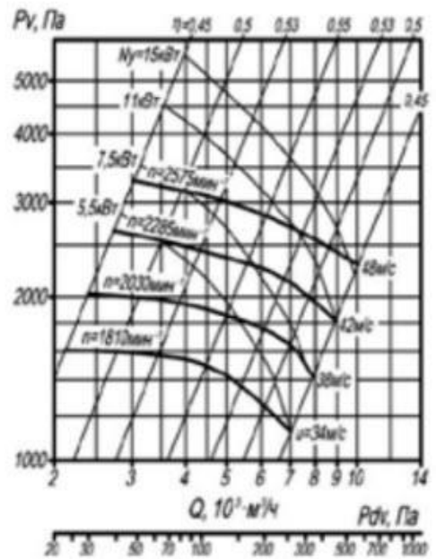
Аэродинамическая характеристика вентилятора ВЦП 7-40 №5 схема 5
